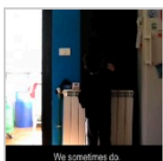
Raya Mazigi
